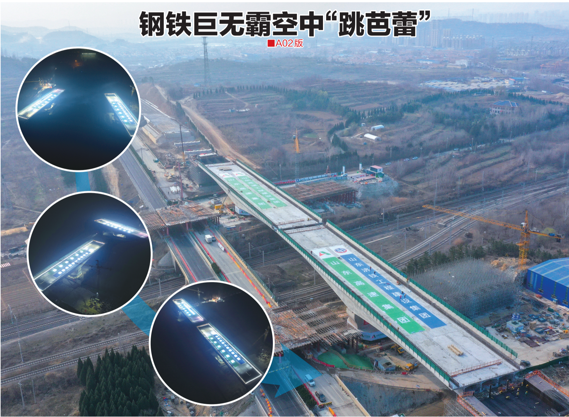
3月24日，荣乌高速烟蓬改扩建项目重要节点——上跨蓝烟铁路转体桥施工顺利完成。两座长度均为122米、单个重量达1.86万吨的转体桥，如“空中芭蕾”般分别完成100.4度和84.8度旋转，与主线实现毫米级对接。 YMG全媒体记者 杨春娜 通讯员 辛扬帆 摄
