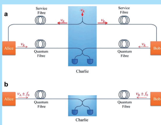
图a为传统闭合光纤架构。图b为中国科学家袁之良团队首创的开放式架构,能够在确保量子通信安全性的同时降低系统建设成本。
