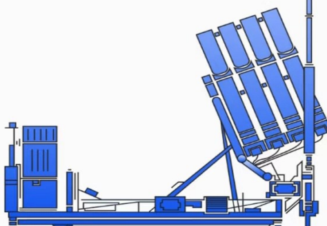
载有20枚“塔米尔”拦截导弹的发射器
