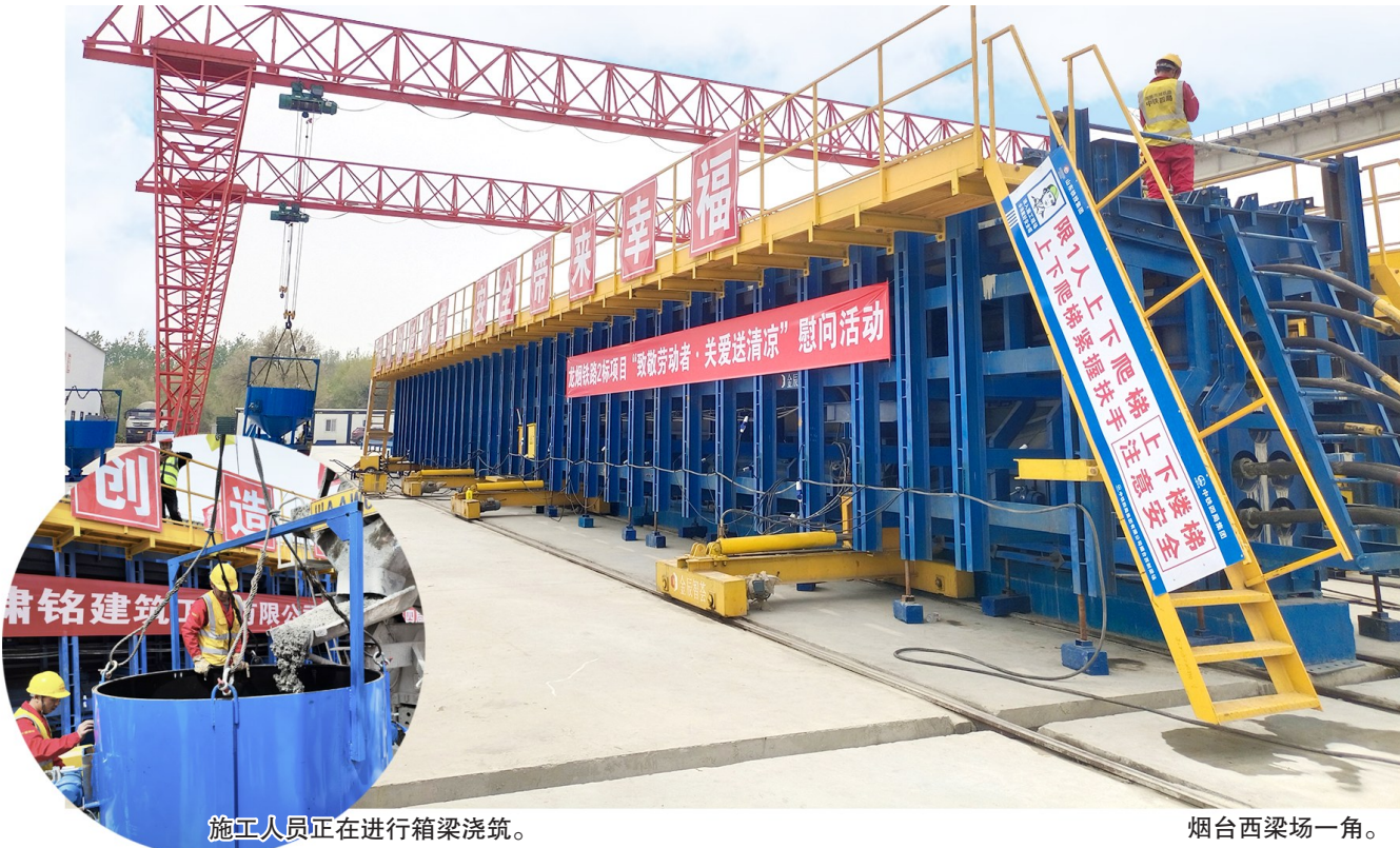
施工人员正在进行箱梁浇筑。
