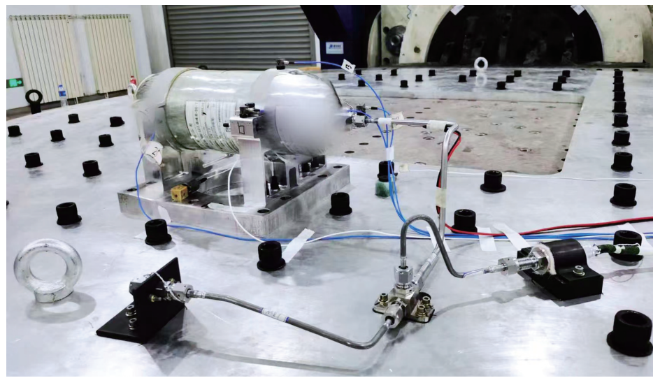
气体推冲系统:高压负载下进行单机振动试验。
