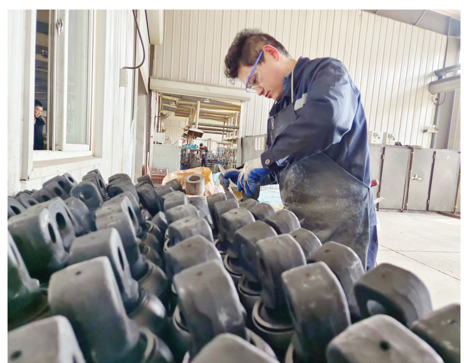
生产车间内,工作人员正在制作推力杆轴承壳。
